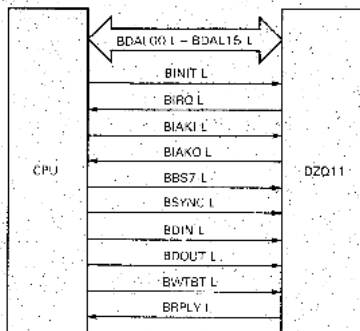
Figure 5-3 DZQ11/Q-bus Interface
