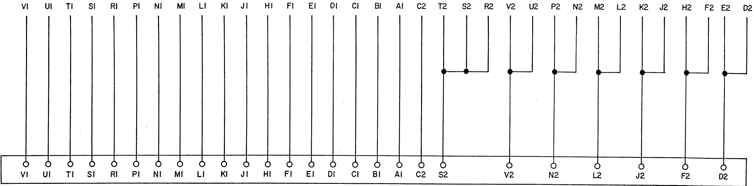
CONNECTOR 7900-0155-0
