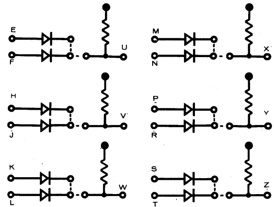
1011 DIODE
