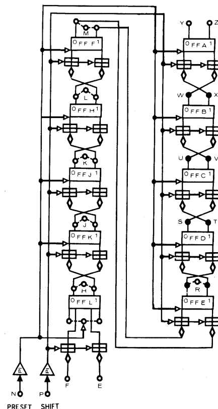
4223 SHIFT REGISTER
