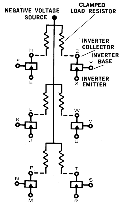
6106 INVERTER
