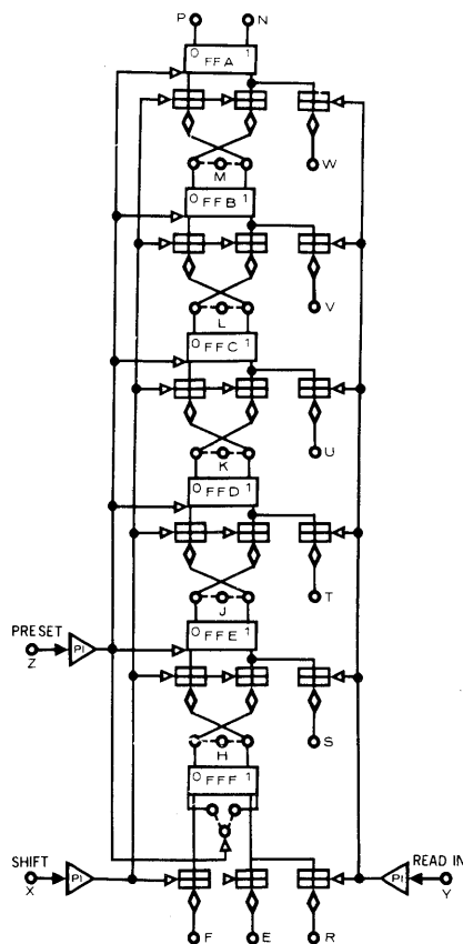
4221 SHIFT REGISTER
