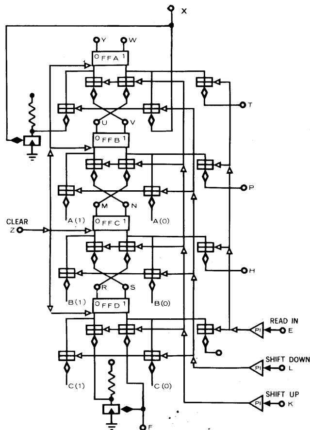
4231 SHIFT REGISTER
