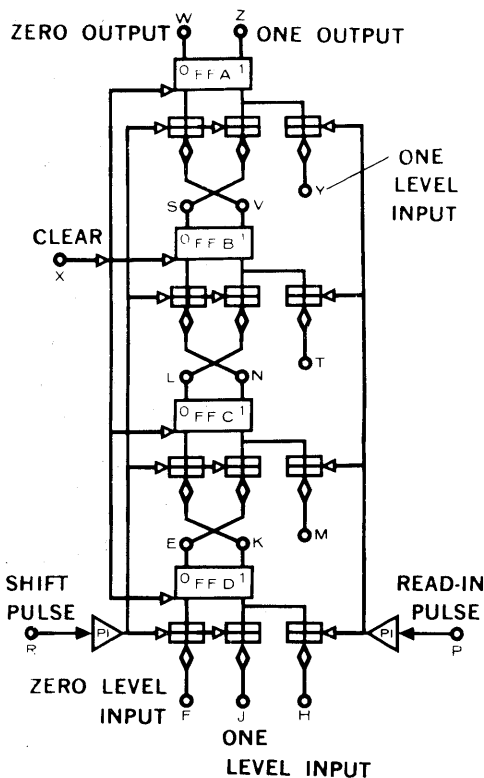
4216 SHIFT REGISTER
