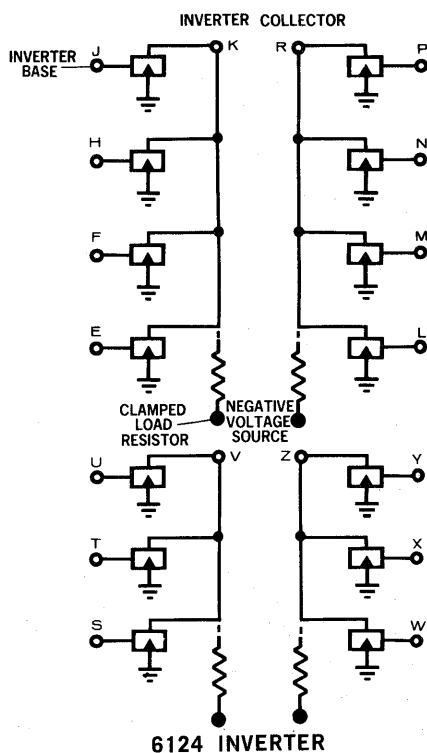
6124 INVERTER
