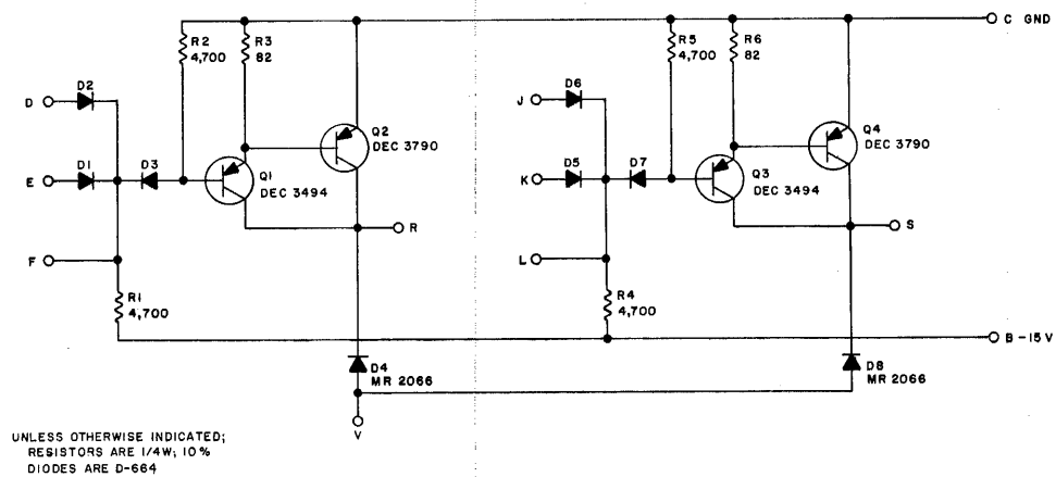
CS-B-W040-0-1 Solenoid Driver W040
