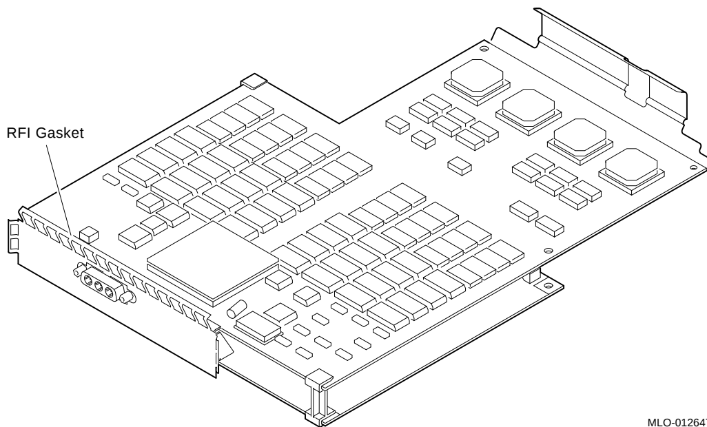
Figure 4–1 SPXgt 24-Plane Graphics Module
